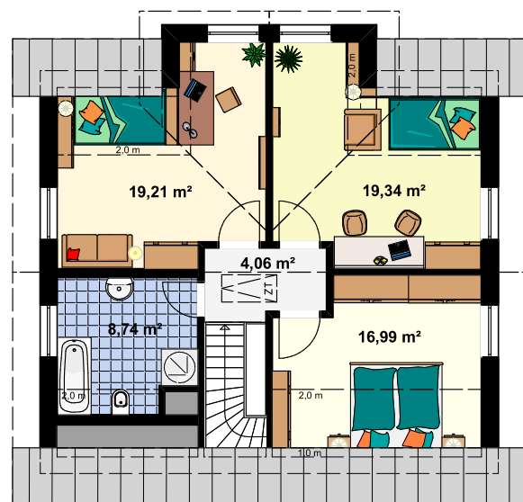
Grundriss Dachgeschoss
