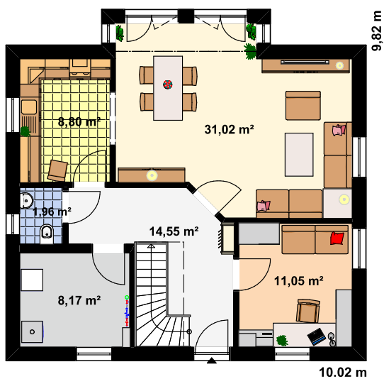
Grundriss Erdgeschoss
